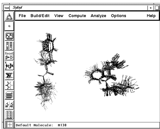
Fig. 3. Two clusters of an actual drug molecule.
